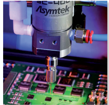
Fig. 1: Asymtek purkštukai
