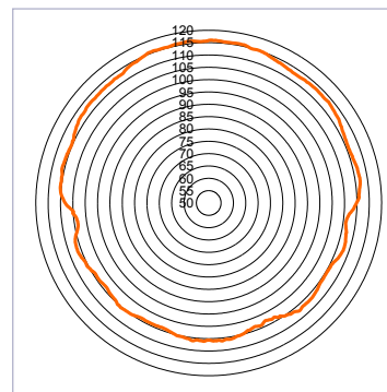
SES2-600-0°, 117 dB(A)
