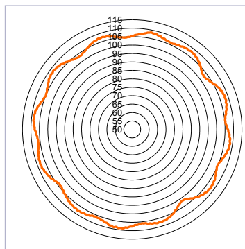
SES2-600-360°, 107 dB(A)
