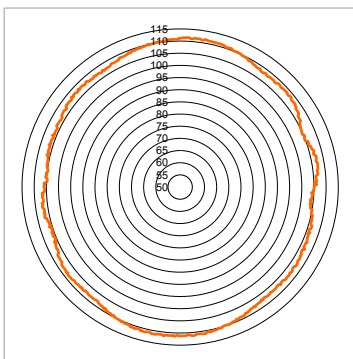
SES2-600-180°, 109 dB(A)
