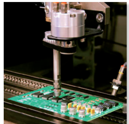
Fig. 2: Revêtement de PCB
