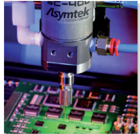
Fig. 1: Machinerie Asymtek
